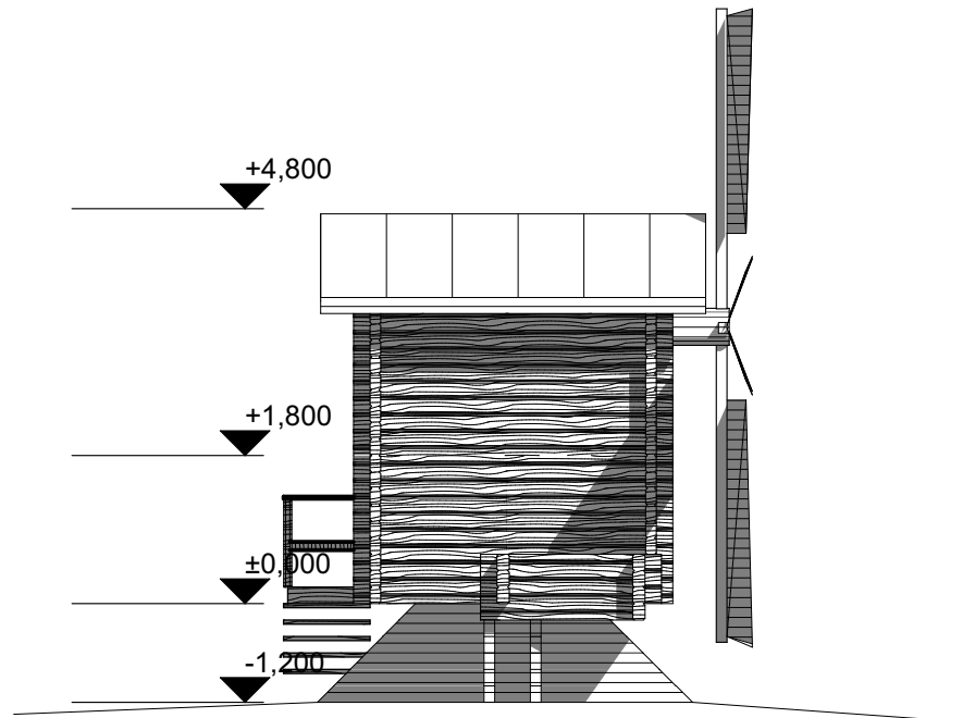
KOILLISEEN 1:100
