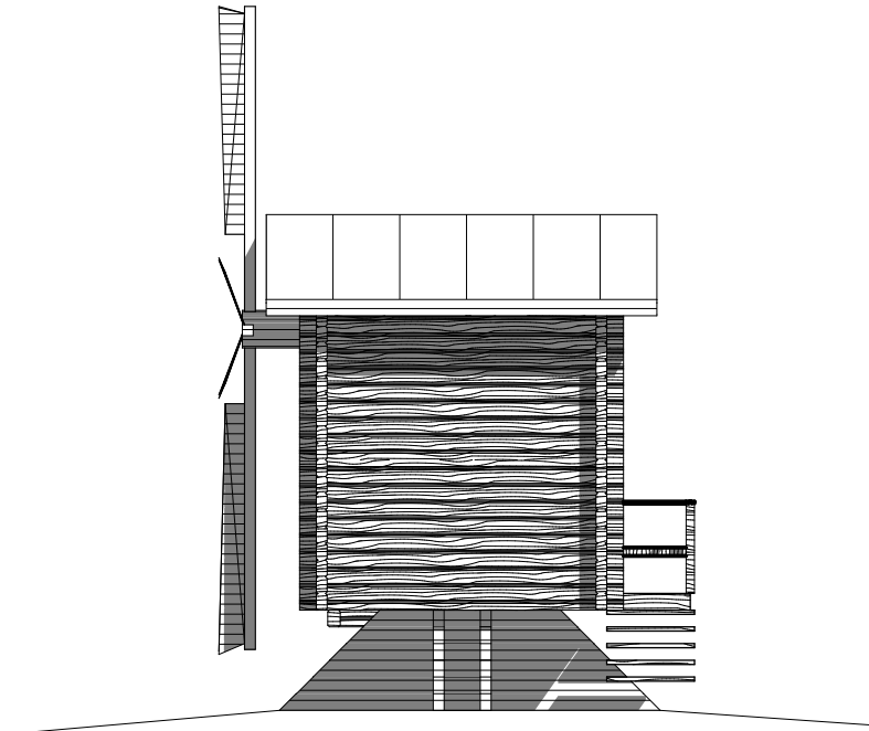
LOUNAASEEN 1:100
