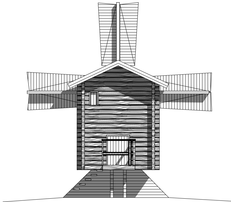
KAARKOON 1:100
