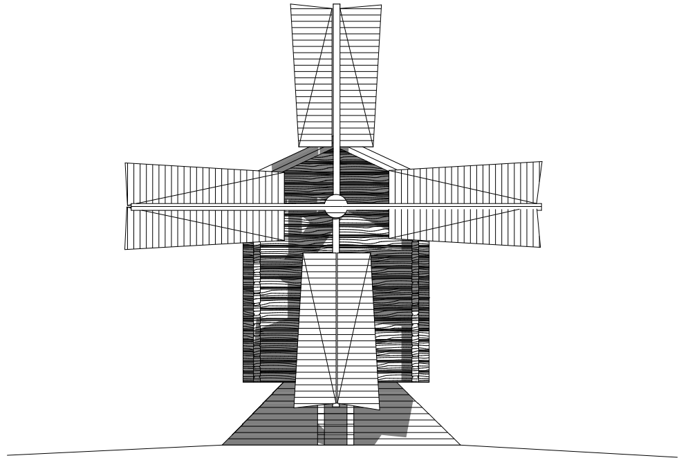
LUOTEeseen 1:100
